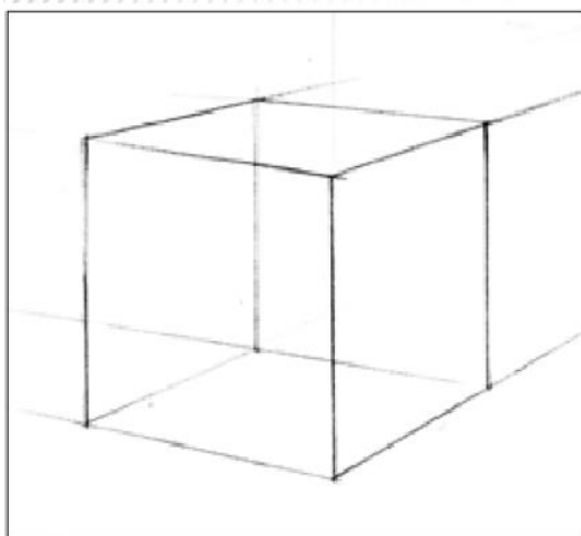
Построение куба
